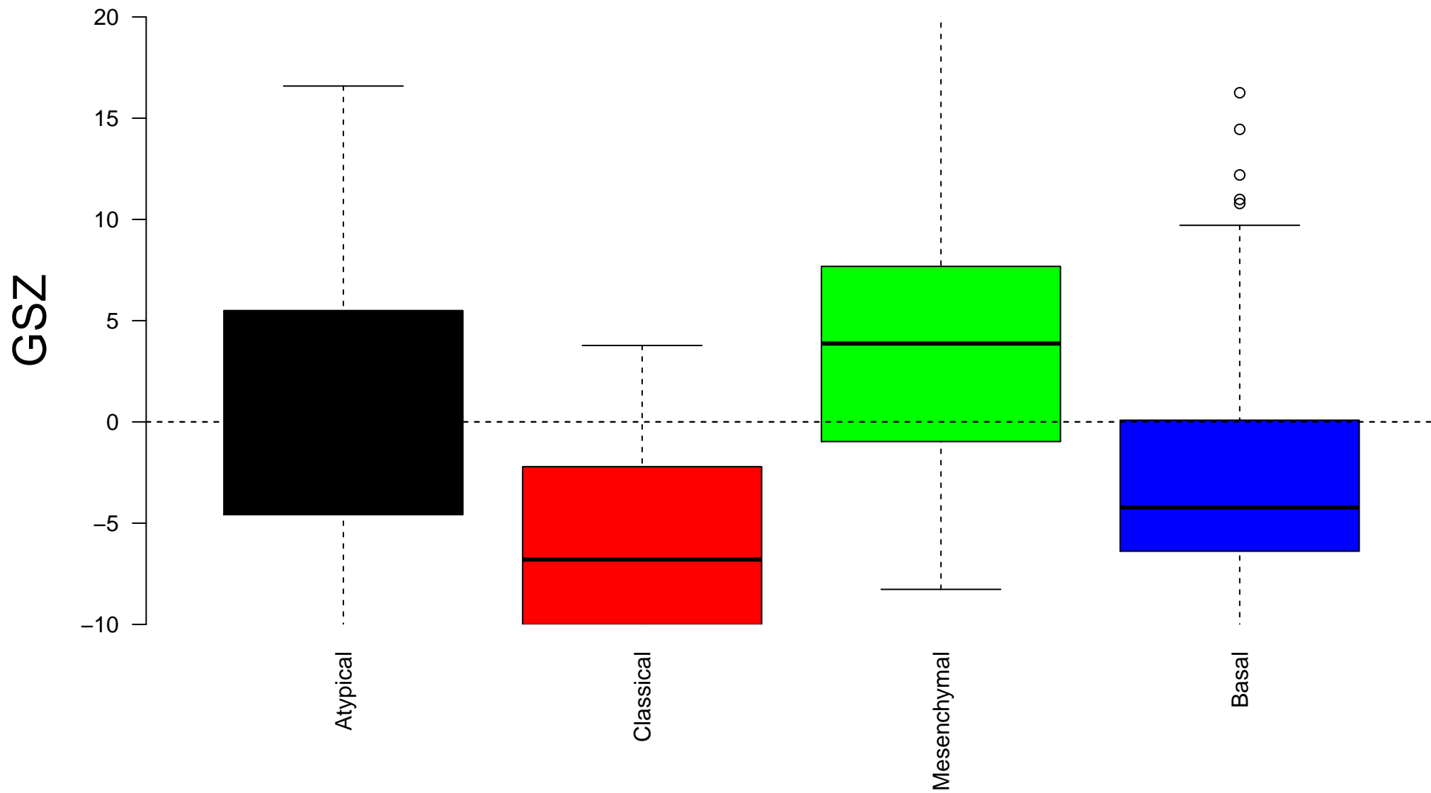
willscher_GBM_Verhaak-MES_expression_B_up
